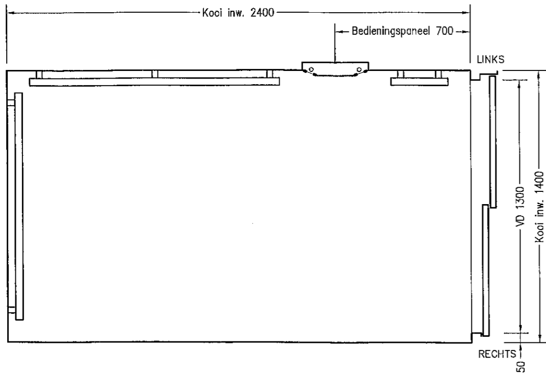
HORIZONTALE KOOIDOORSNEDE
